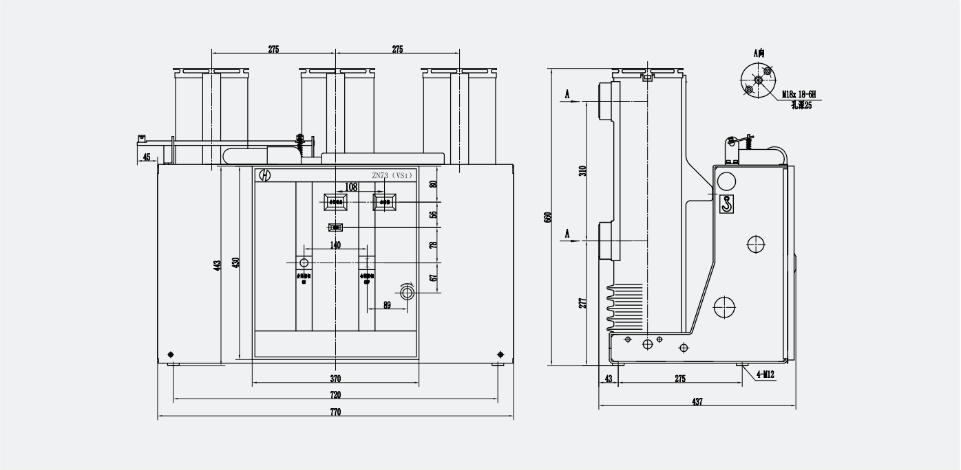
6.2 固定式真空断路器外形尺寸图
