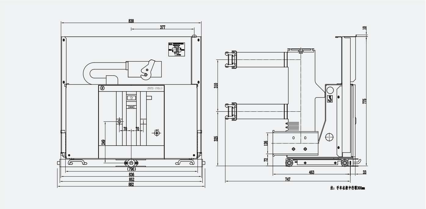
6.1 手车式真空断路器外形尺寸图
